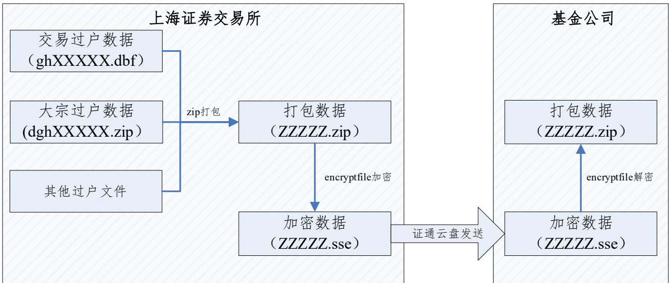
图 4：基金公司接口数据流图
